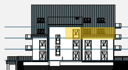
pohled severozápadní
